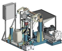
Установка сухого растаривания (пластиковые барабаны)
