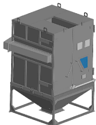
Модуль растаривания биг-бэгов закрытого типа, без ГПМ
